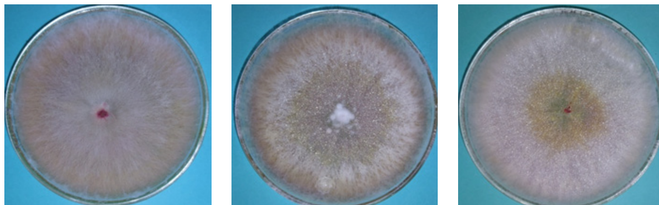
F. semitectum 1
